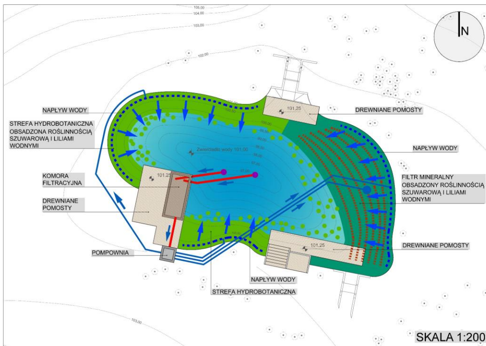
FILTR MINERALNY/STREFA HYDROBOTANICZNA OBSADZONY ROŚLINNOŚCIĄ SZUWAROWĄ
